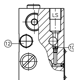
Type PSV.../D...-2
